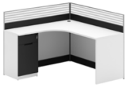
型号: 20-LP4712 工位 尺寸: 1220W*1220D*1050H(mm) 型号: 20-LP4814 工位 尺寸: 1420W*1420D*1050H(mm)
